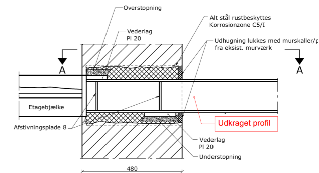
Lodret snit
