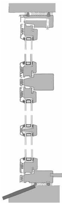
Termovindue, alu/træ
