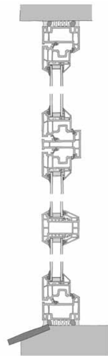
Termovindue, plast
